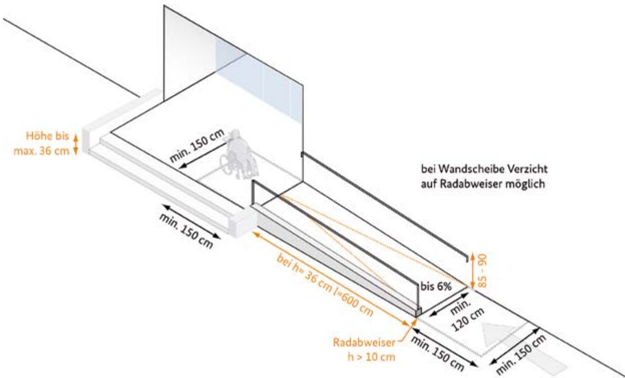
Standardaufbau Rampe – die Weiterführung der Radabweiser und Handläufe über die Länge der Rampe hinaus ist nicht erforderlich
